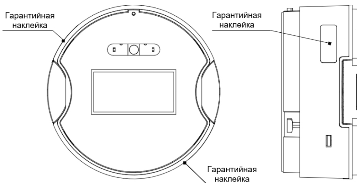
Рисунок 17 - Расположение гарантийных наклеек на электронном модуле газоанализатора
