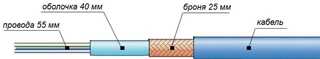
Рисунок 21 – Подготовка кабеля с бронезащитой
