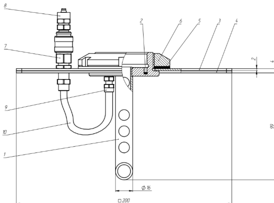
Рисунок 30 - Общий вид комплекта.
